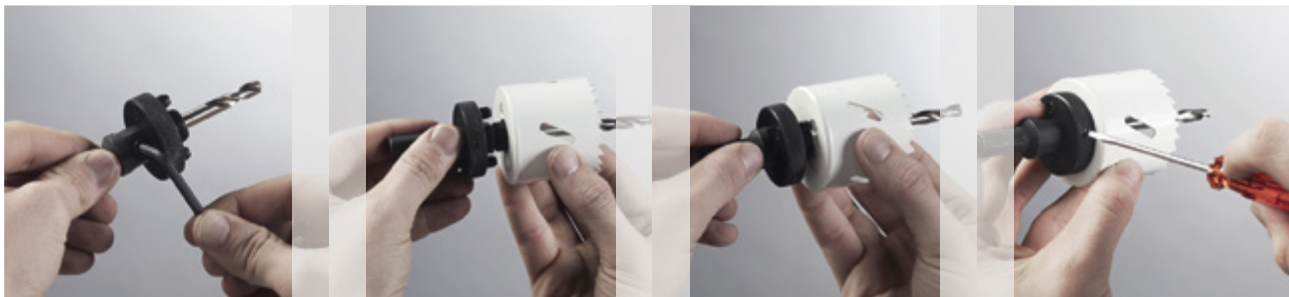
הכנסת מקדח המרכז. הידוק באמצעות בורג אלן.
